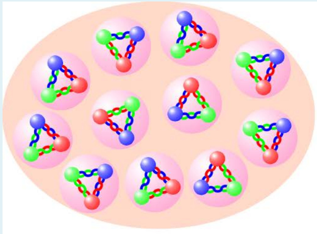
通常物質
