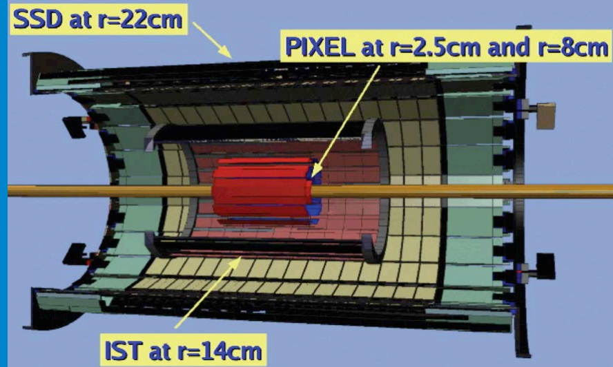
STAR HFT
