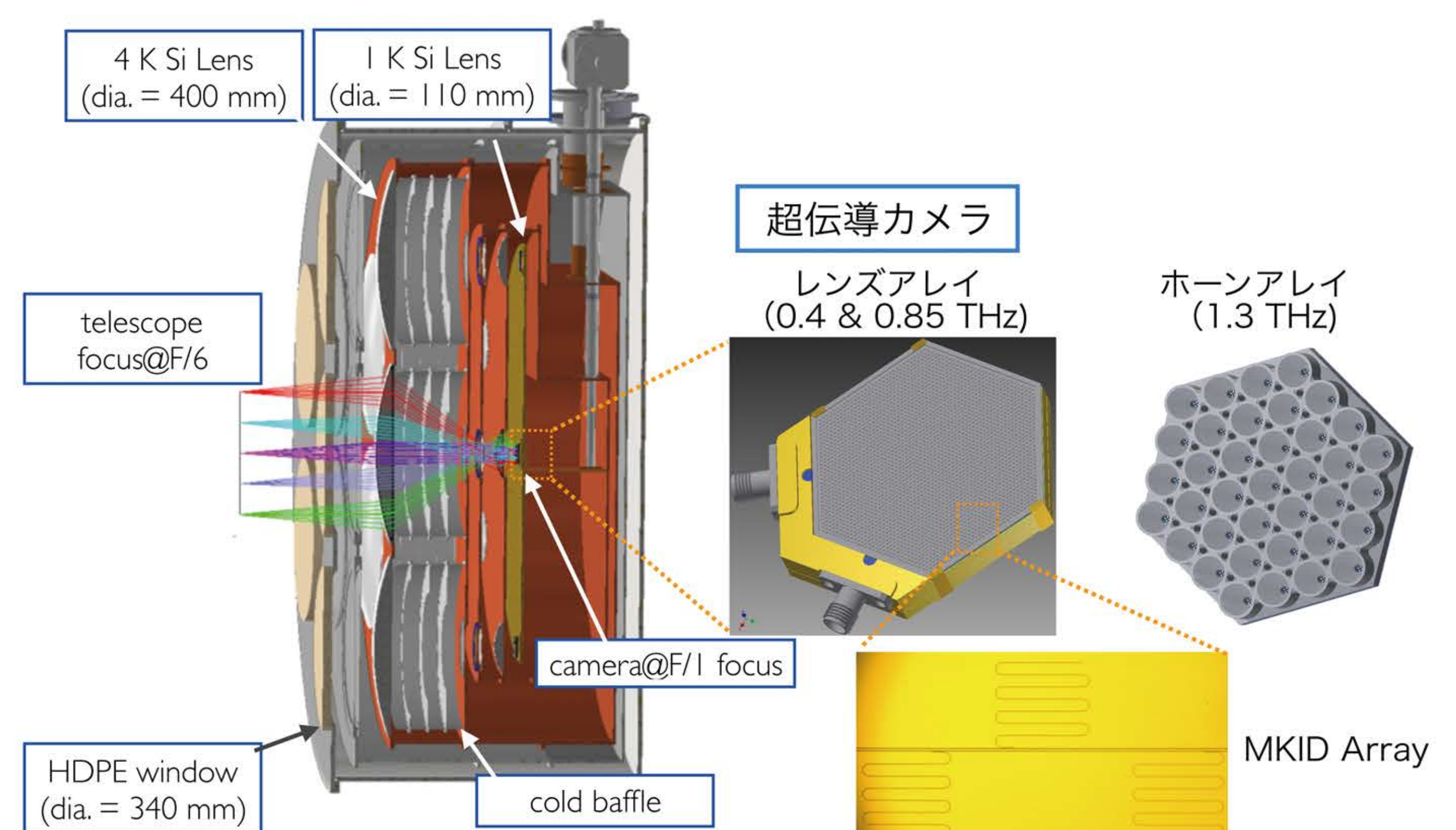
図11 MKIDと平面アンテナ
