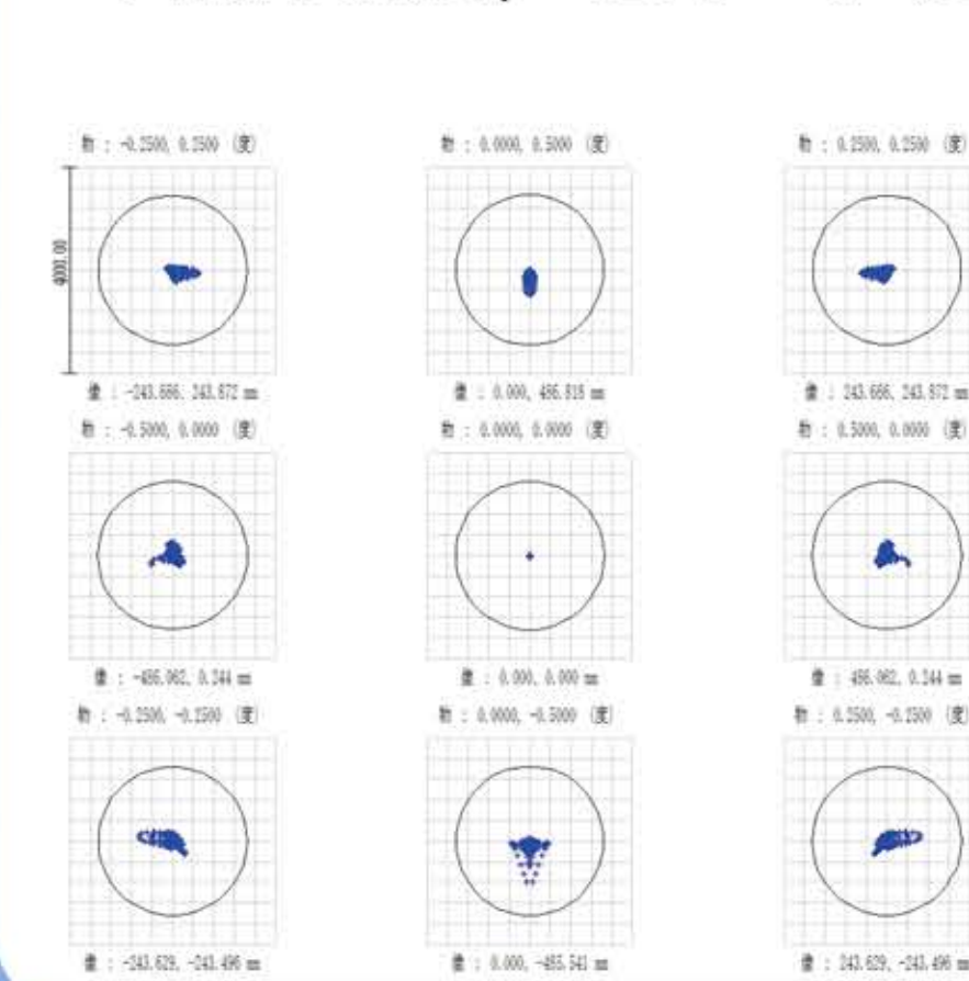
←図10 光線解析ソフトZEMAXによる像面スポットダイアグラム評価
