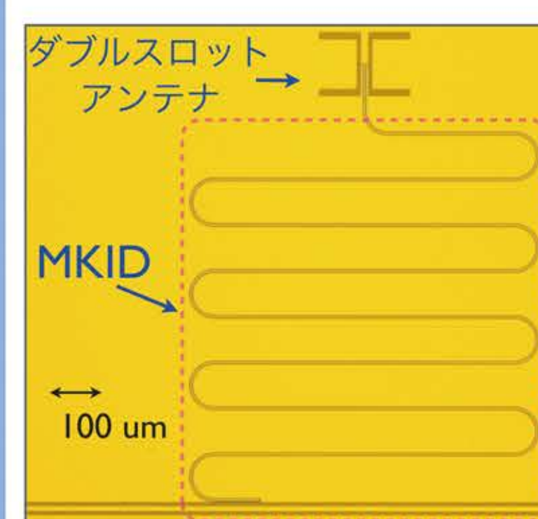
図11 MKIDと平面アンテナ
