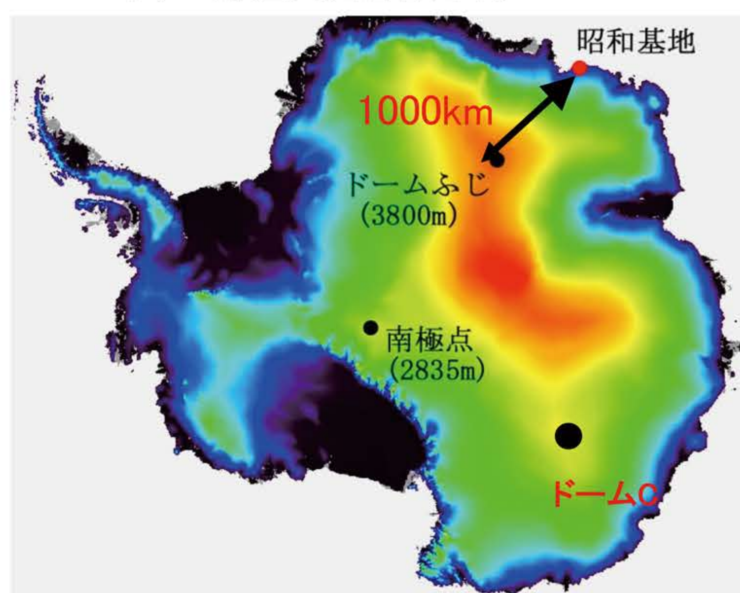
図2 南極大陸と各基地
