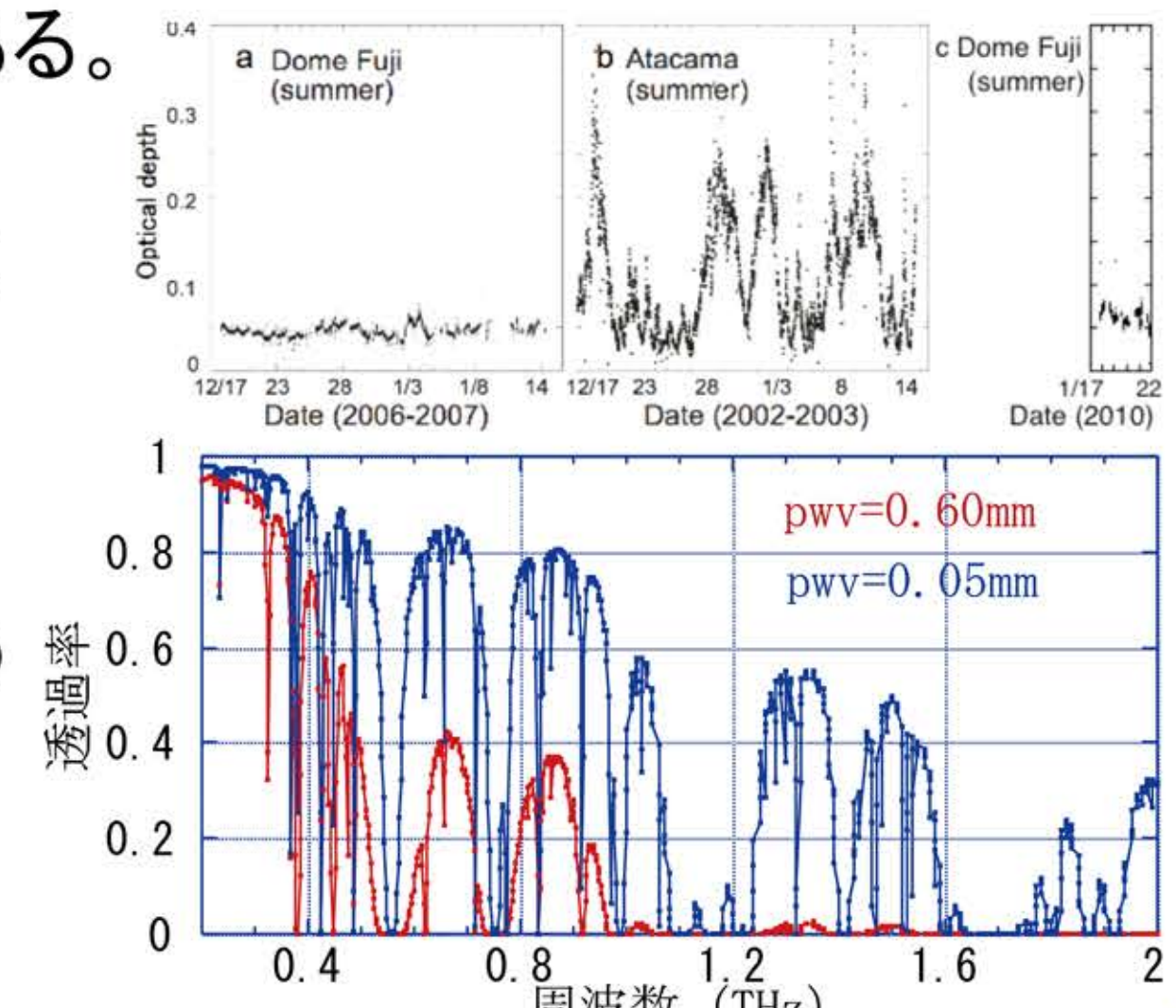
図5→ 大気透過率の予想値
